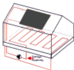
Ηλιακοί συλλέκτες και ενδοδαπέδιο σύστημα θέρμανσης με μια βοηθητική πηγή θέρμανσης (π.χ. κεντρική θέρμανση).
